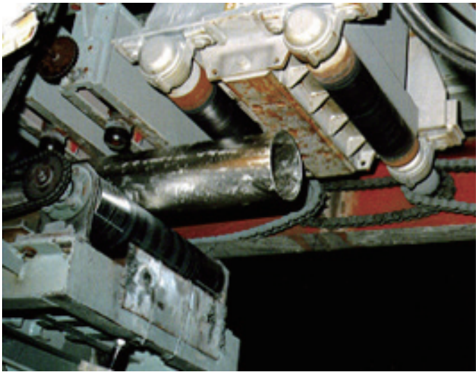
自動引き上げによる鋼管のめっき
